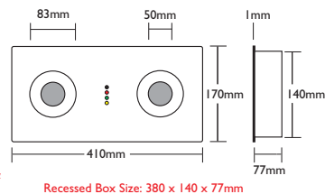
"CRYSTALITE" Cat. CE-DPC-2X3W-12V-GC-2H & CE-DPC-2X3W-12V-GC-3H
